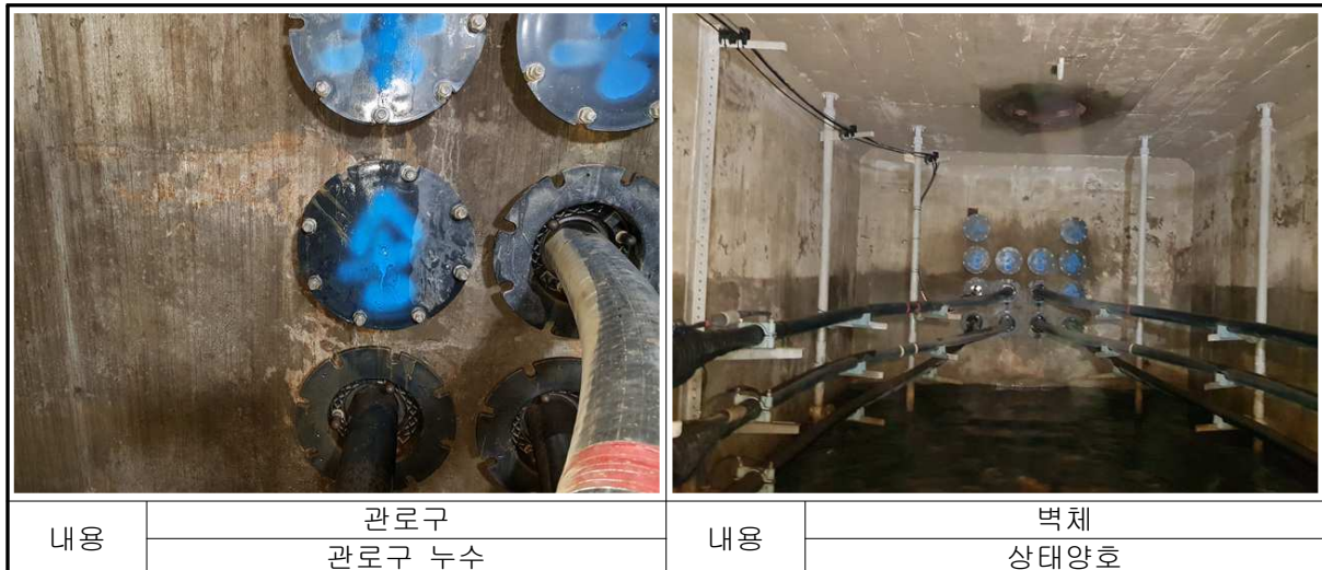
【사진 1.34】 맨홀 내부 주요 손상
