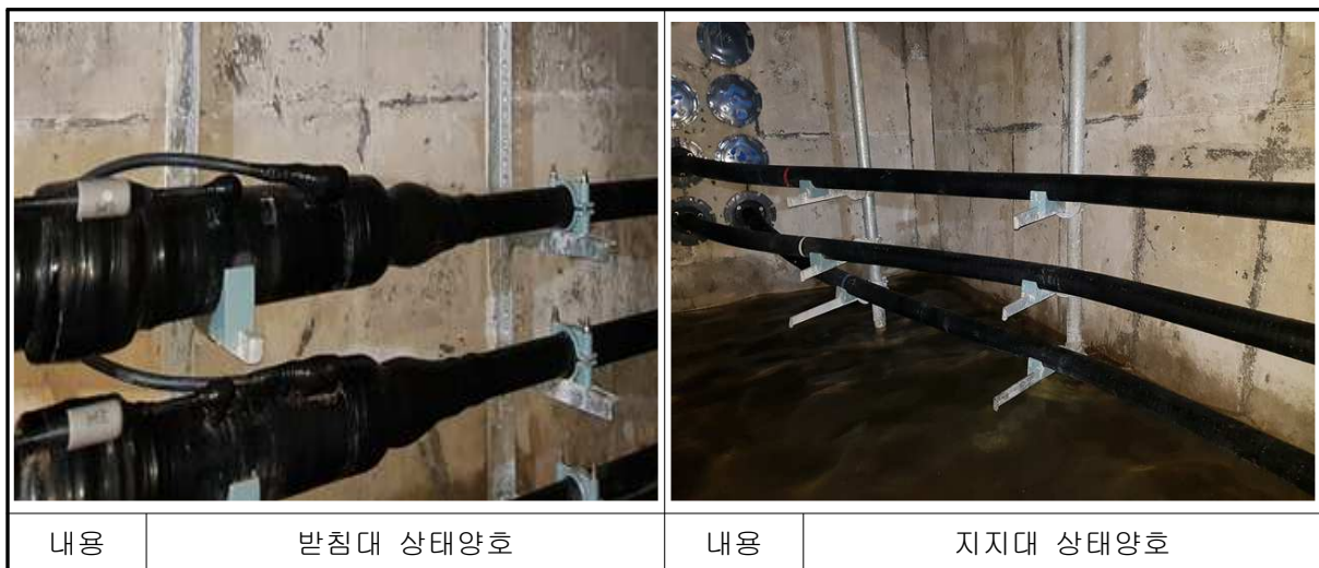
【사진 1.32】 부속 및 부대설비 현황
